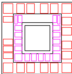
Metal. chłodz. termoel. - widok z góry Metalized TEC - top view
